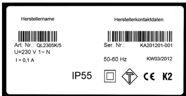
Bild 5-2: Typenschild mit CE-Kennzeichen und Herstellerkennzeichnung
